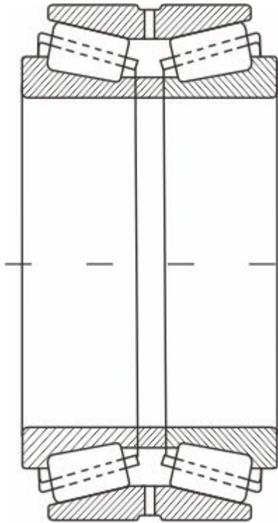
图 Design 12
